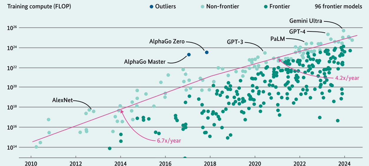
Rechenaufwand für das Training von Frontier-Modellen
